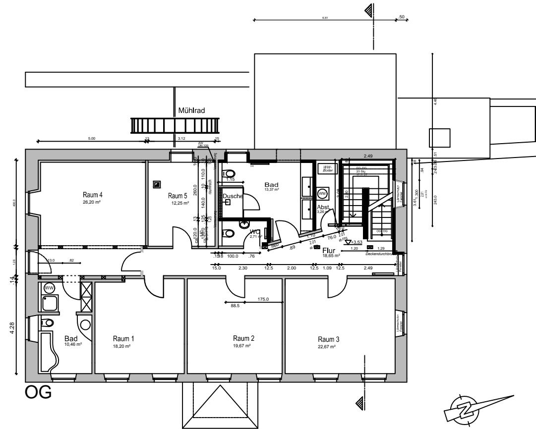
OBERGESCHOSS GRUNDRISS
