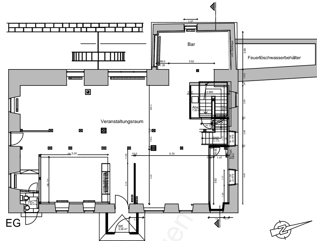
ERDGESCHOSS GRUNDRISS
